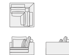
Corner W1080 D1080 H850 SH400
