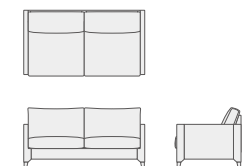
2P W1600 D870 H780 SH400
