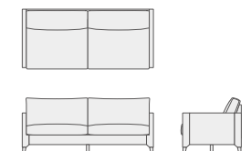
3P W1900 D870 H780 SH400
