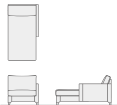
One arm couch W800 D1470 H780 SH400
