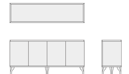
1700 4 doors W1700 D450 H800
